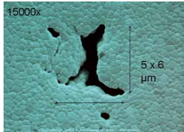
Abbildung 6 Fehlerhaft gepresstes ZrO_2 , REM 15.000fach vergrößert. Die Dauerbiegebruchfestigkeit ist erheblich eingeschränkt.
